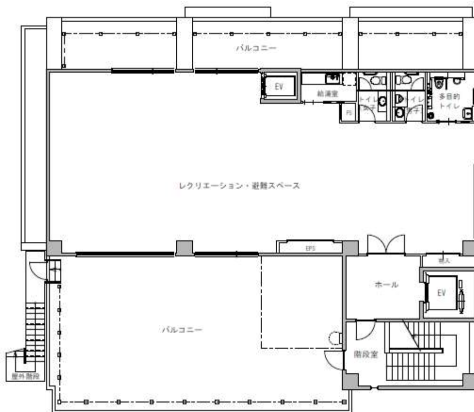
2階平面図
