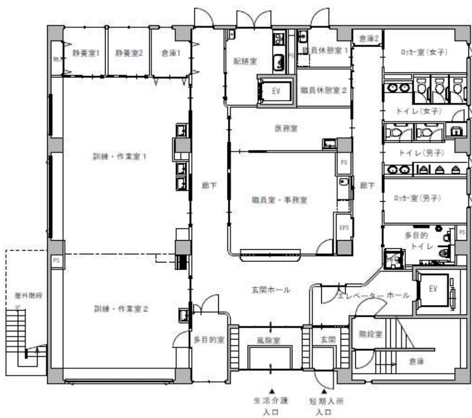
1階平面図
